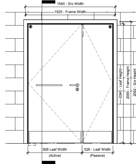
03 Push Face 1 : 25
