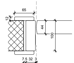
07 Jamb Detail 1 : 5
