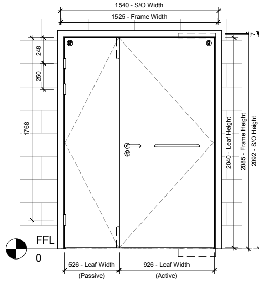
02 Pull Face 1 : 25
